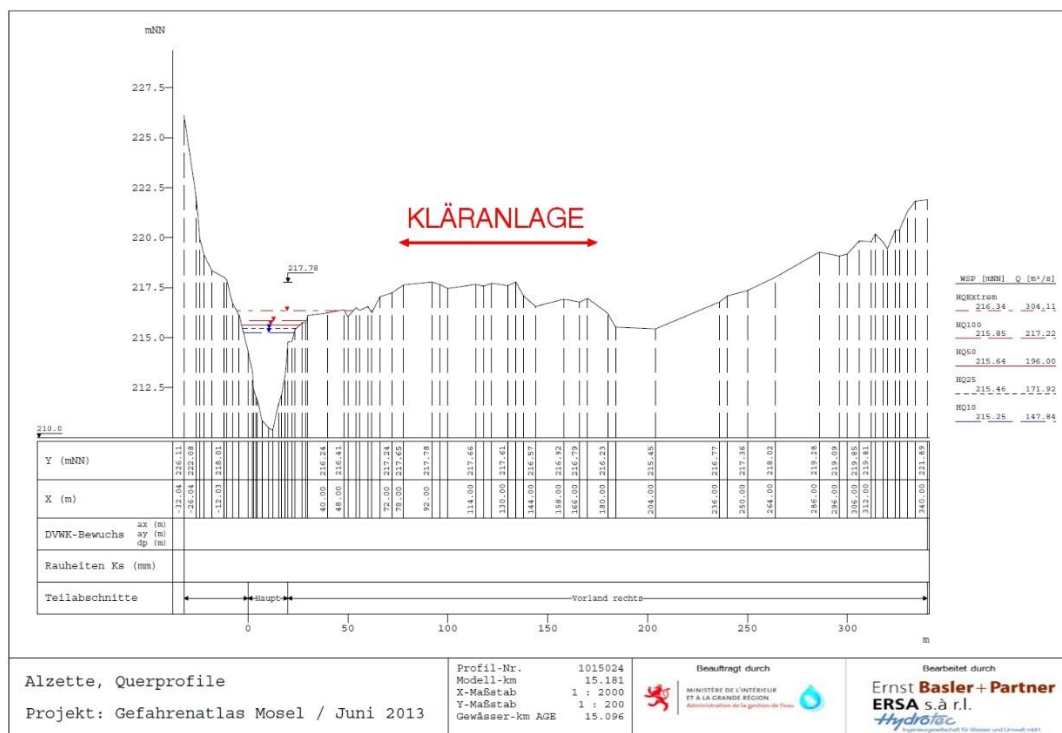
Abbildung 63: Kläranlage Beringen
