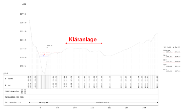
Abbildung 63: Kläranlage Beringen
