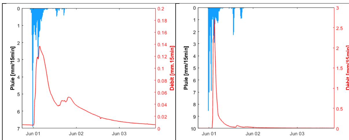
Abbildung 30: [Links] Niederschlag und Abfluss der Weißen Ernz an der Larochette vom 31. Mai bis 3. Juni 2018. [Rechts] Niederschlag und Durchfluss des Hallerbachs vom 31. Mai bis 3. Juni 2018.
