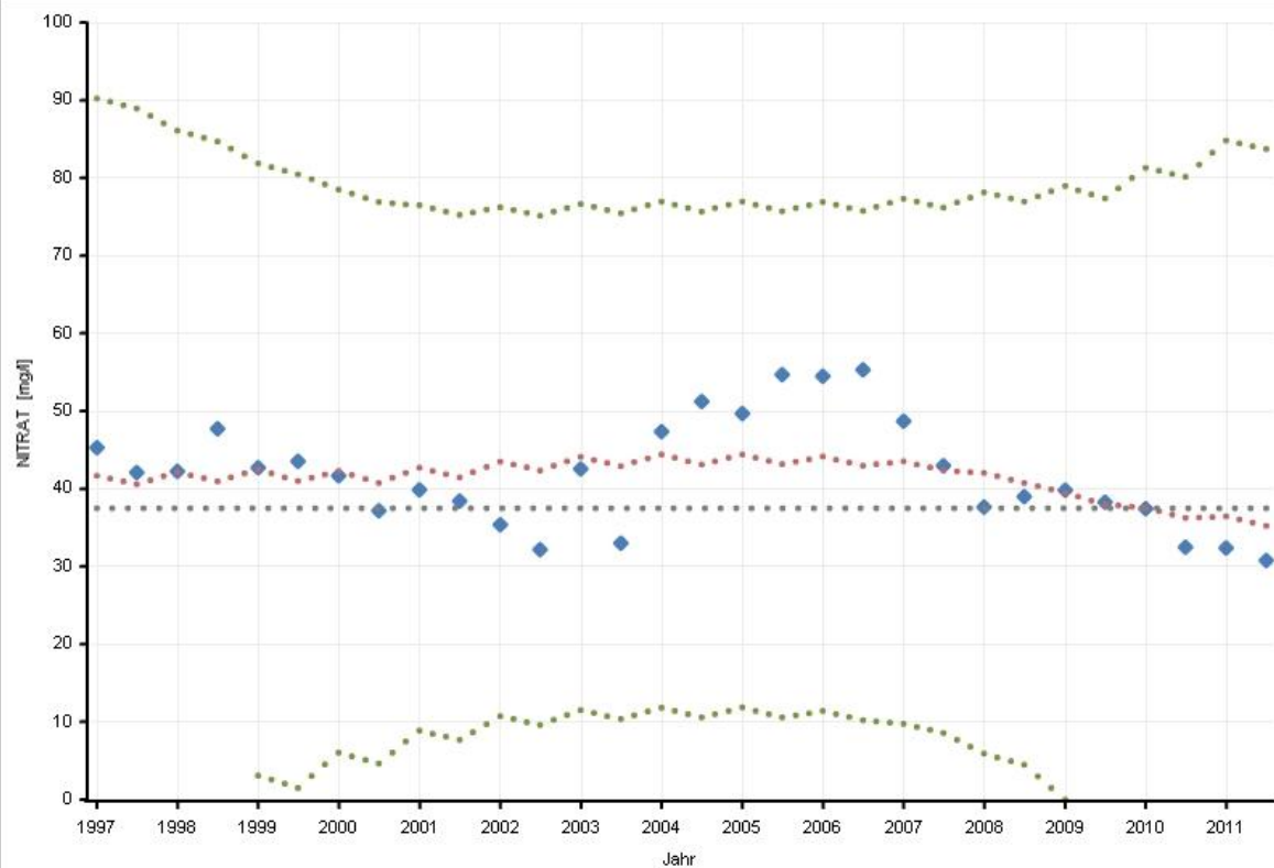
Smoother und Vertrauensbereich für Parameter G154 im Grundwasserkörper Leibnitzer Feld [MUR] (GK100098)
