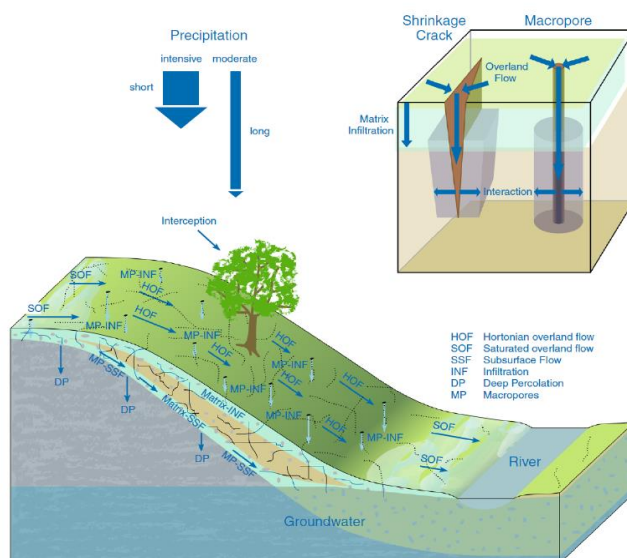
Abbildung 46: Abflussbildungsprozesse nach Steinbrich et al. (2016)
