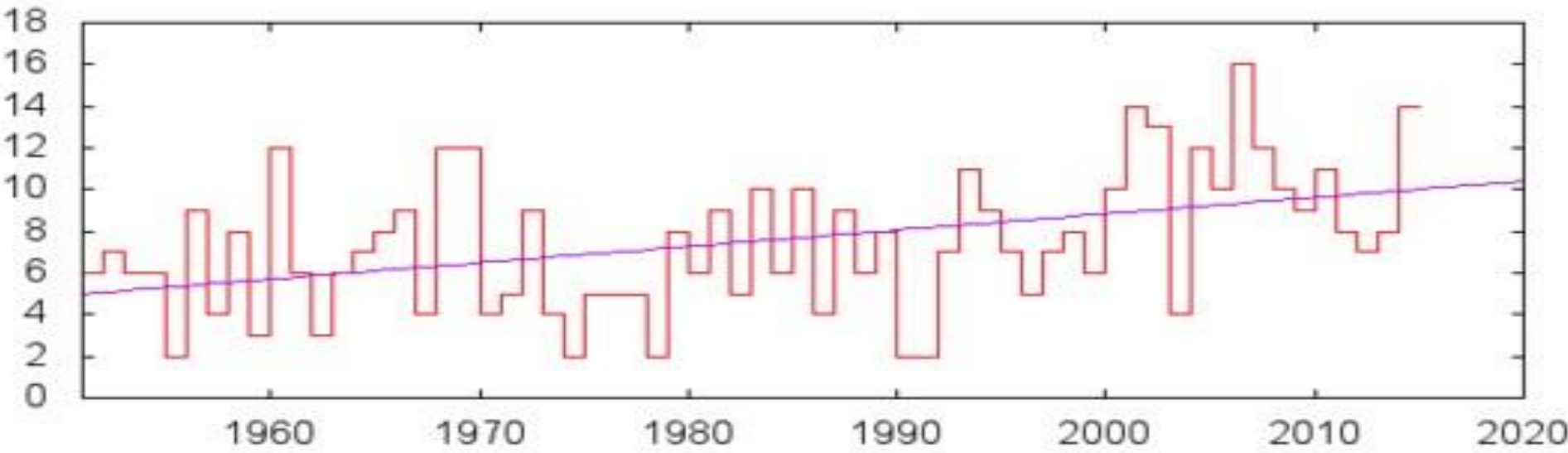
Anzahl Tagen mit mehr als 50 mm/Tag oder mehr pro Jahr
